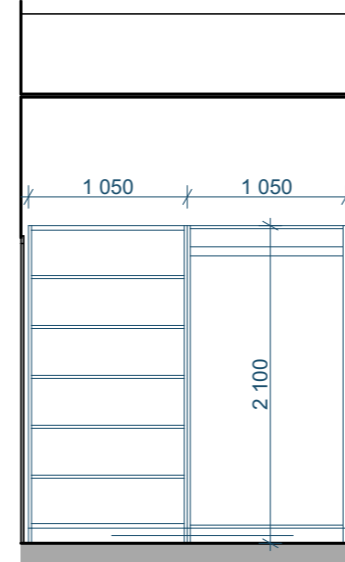
105 04 1:50
